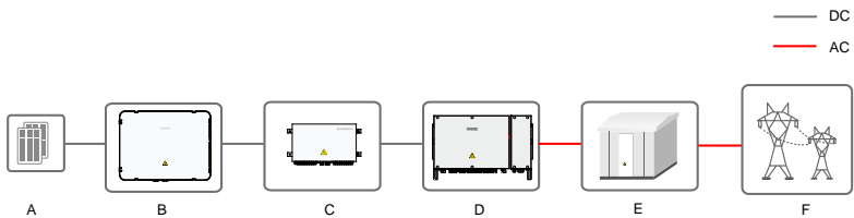
Figura 3-1 Composición del sistema de generación FV conectado a la red
