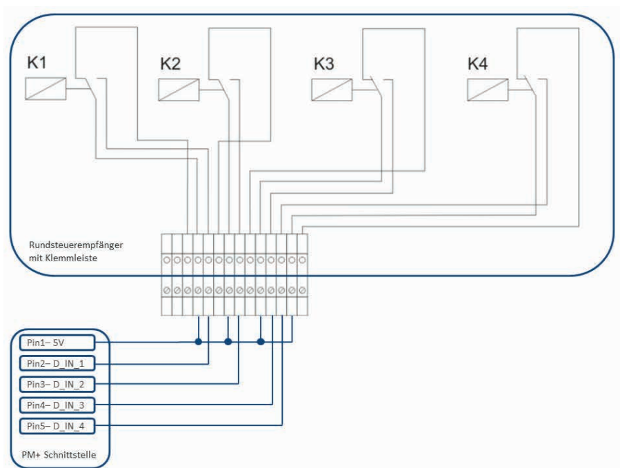
Abb.: Schematische Darstellung eines Rundsteuerempfängers mit vier Relais.
