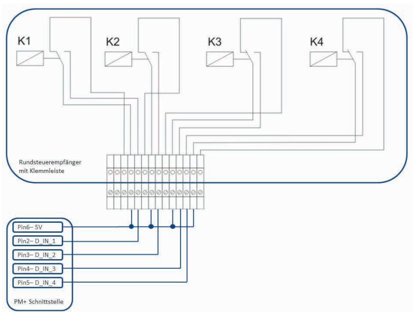
Abb.: Schematische Darstellung eines Rundsteuerempfängers mit vier Relais. Diese Relais sind für die Blindleistungsregelung mit der PM+ Schnittstelle verdrahtet.
