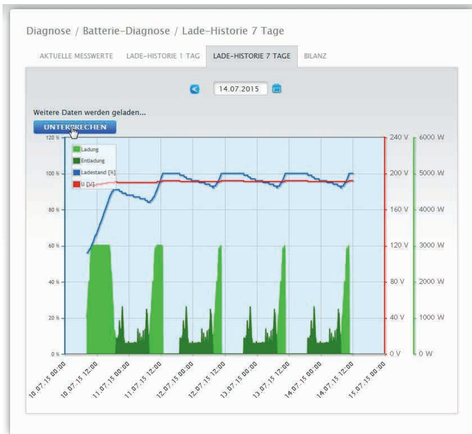
Abb.: Batterie-Diagnose - Lade Historie 7 Tage
