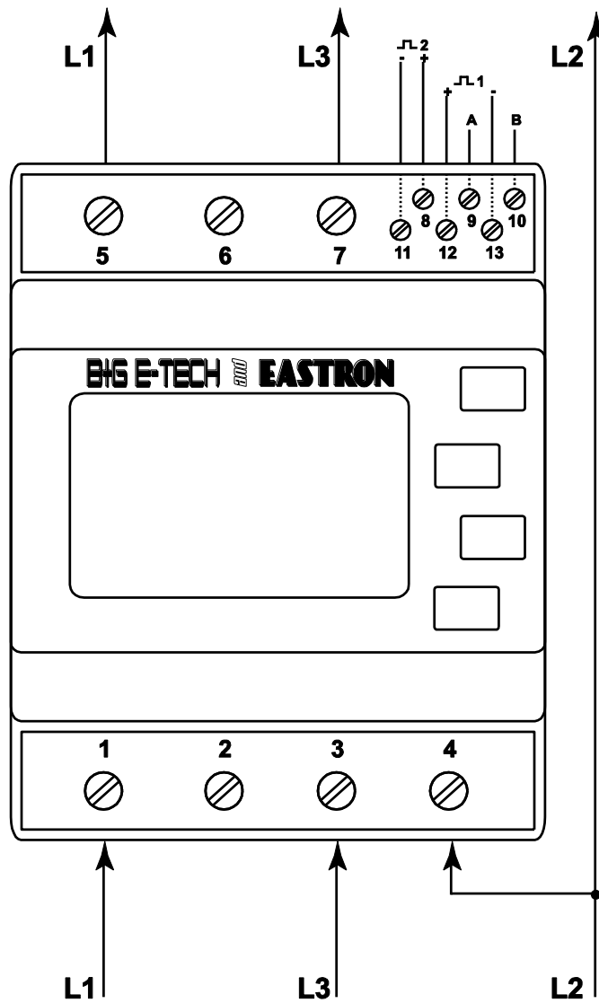
Anschlussbild dreiphasiges System ohne Neutralleiter (3p3)
