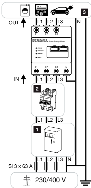
Afb.: Aansluitvoorbeeld voor directe meting van stroomsterktes
