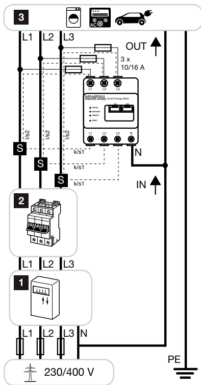
Fig.: Esempio di collegamento per la misurazione indiretta dell'intensità di
