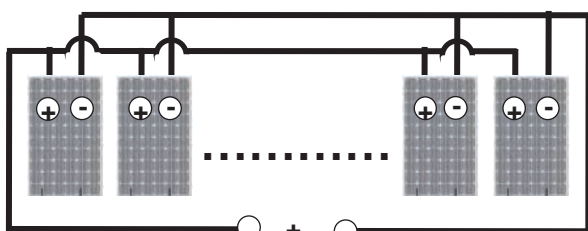
Collegamento in parallelo per ottenere valori di corrente superiori
