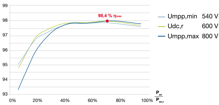
PIKO CI 100
