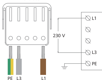
IT monofase
