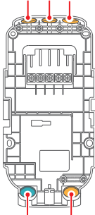
Ingresso del cavo per le comunicazioni
