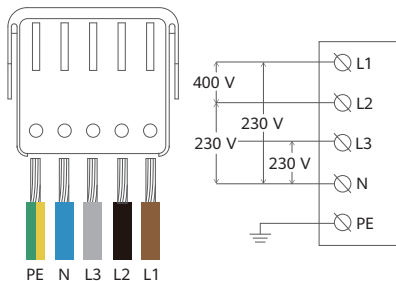
TN e TT trifase
