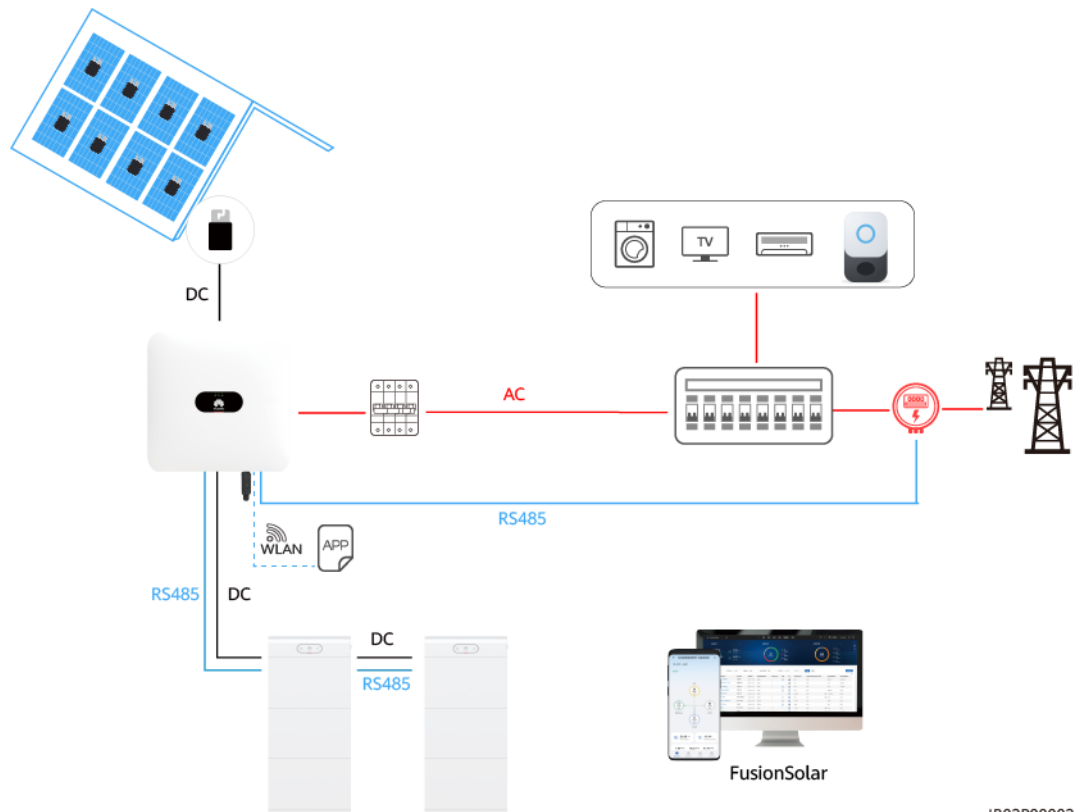
Abbildung 2-7 Netzgekoppeltes Szenario
