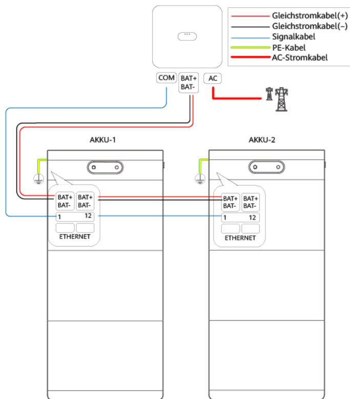
Abbildung 3-1 Kabelverbindungsplan
