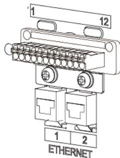
Abbildung 5-5 Signalanschluss
