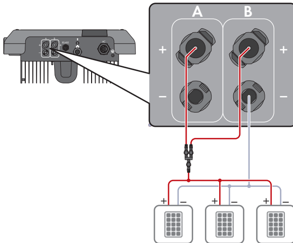
Afbeelding 8: Overzicht van de aansluiting bij parallelschakeling van de DC-ingangen A en B
